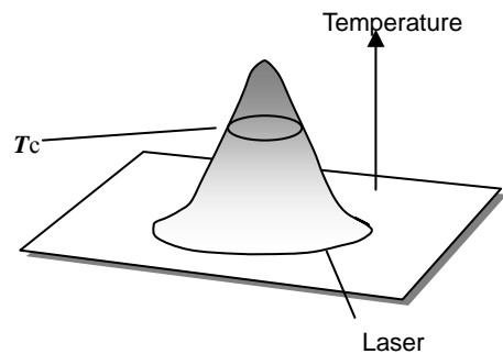
図.10 レーザスポットと温度分布
