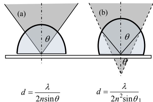
図 13 (a)半球 SIL と (b)超半球 SIL
