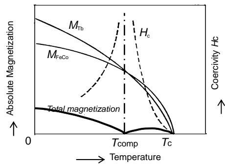
図 8 TbFeCo の副格子磁化の温度変化
