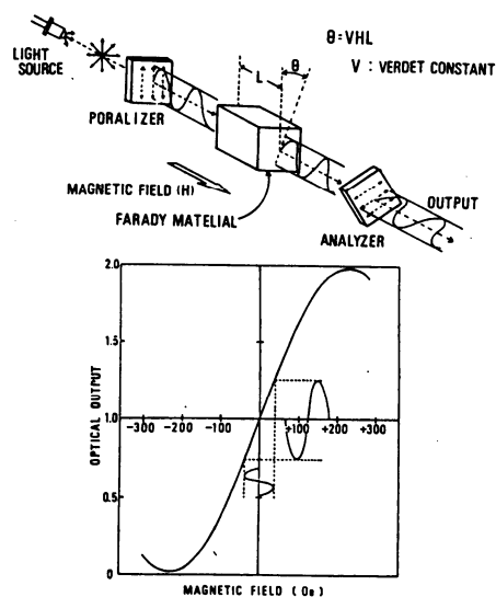
図. 17 電流磁界センサの原理図
