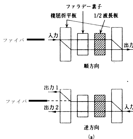
図 16 偏光無依存アイソレータの構成図
