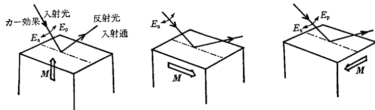
図2 磁気カー効果
